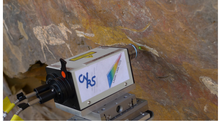
Fig. 4. Spectroscopie Raman portable utilisée pour identifier des pigments sur un site de peinture rupestre. Lieu : site de Maloti-Drakensberg, Afrique du Sud, inscrit au Patrimoine mondial. (Photo © L. Ronat.)
