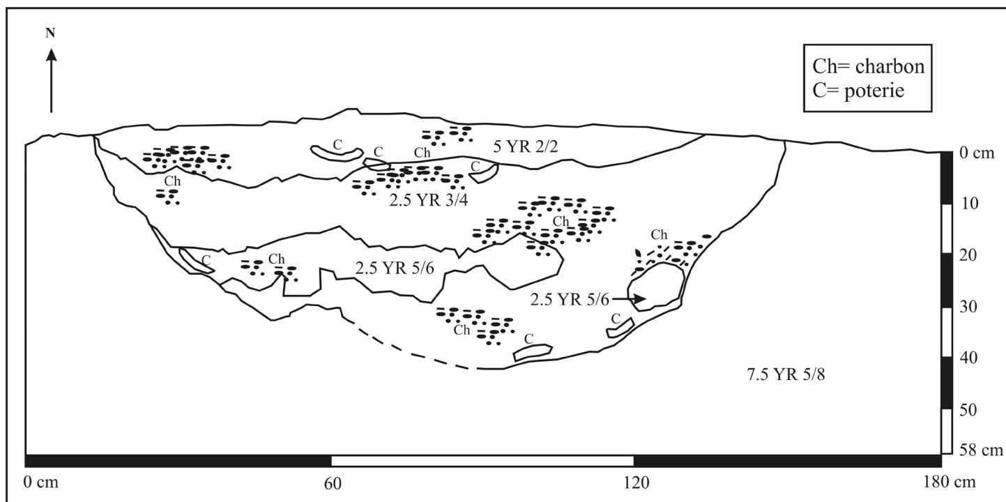
Fig. 10. Relevé d'une coupe à l'échelle 1/10.
